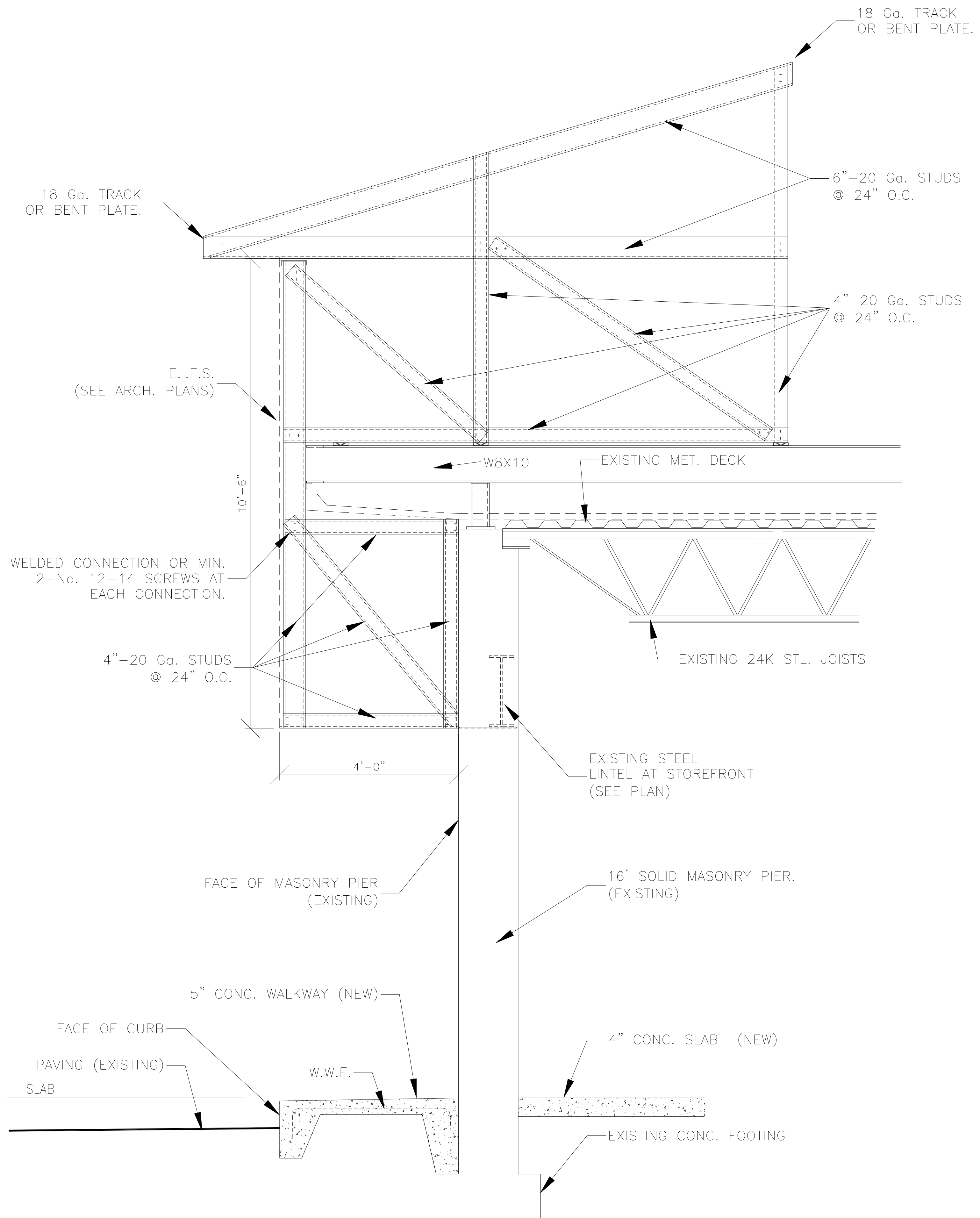
SECTION - 1 SCALE: 3/4"=1'-0"
